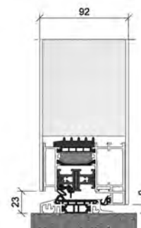
KÖSTER ADVANCE 108 optionale Ausführung mit schrägem Blendrahmen
